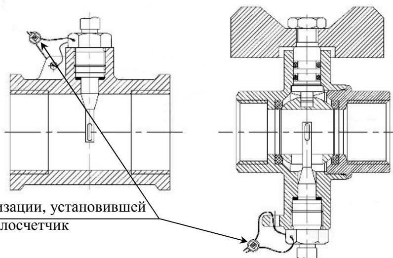
Рисунок 4 - Схемы пломбировки термопреобразователя сопротивления на трубопроводе
