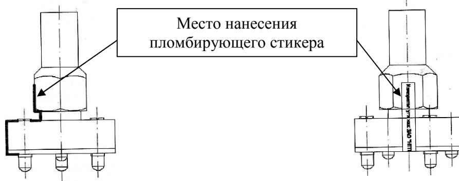
Рисунок 2.1 - Схема пломбировки от несанкционированного доступа измерителей (вид сбоку)
