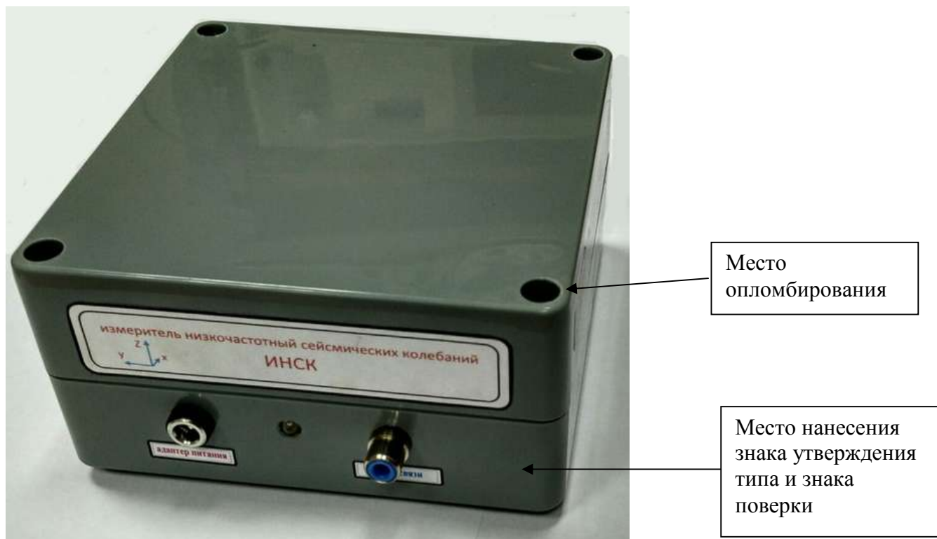
Рисунок 1 - Внешний вид измерителей низкочастотных сейсмических колебаний ИНСК
