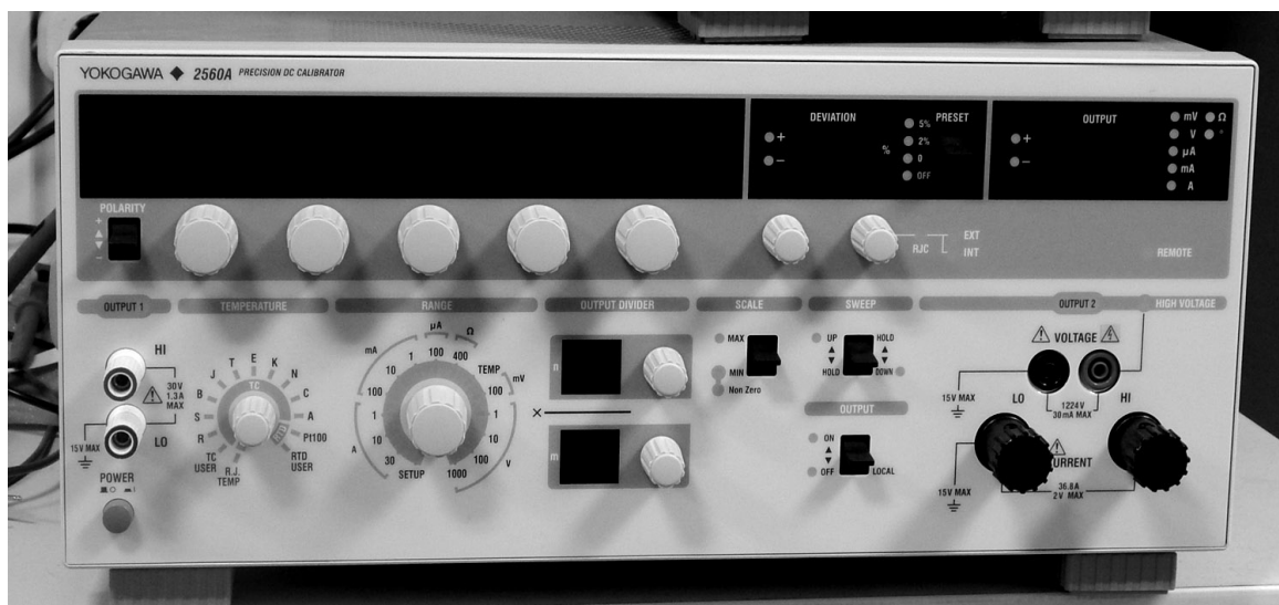
Рисунок 1 - Внешний вид источников напряжения и силы постоянного тока эталонных 2560А
