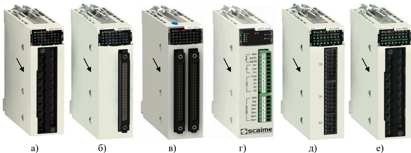
Рисунок 1 - Общий вид модулей а) VMXAMxxxxxu и VMEANxxxxxu, б) VMXART0414y, в) VMXART0814y, г) PMESWT0100, д) VMXENC0200y, е) VMXENC0800y (х: цифра, у: отсутствие символа – базовое исполнение; символ «Н» – исполнение с повышенным уровнем защиты, символ «С» – исполнение с защитным покрытием (лак) от химически агрессивных сред
