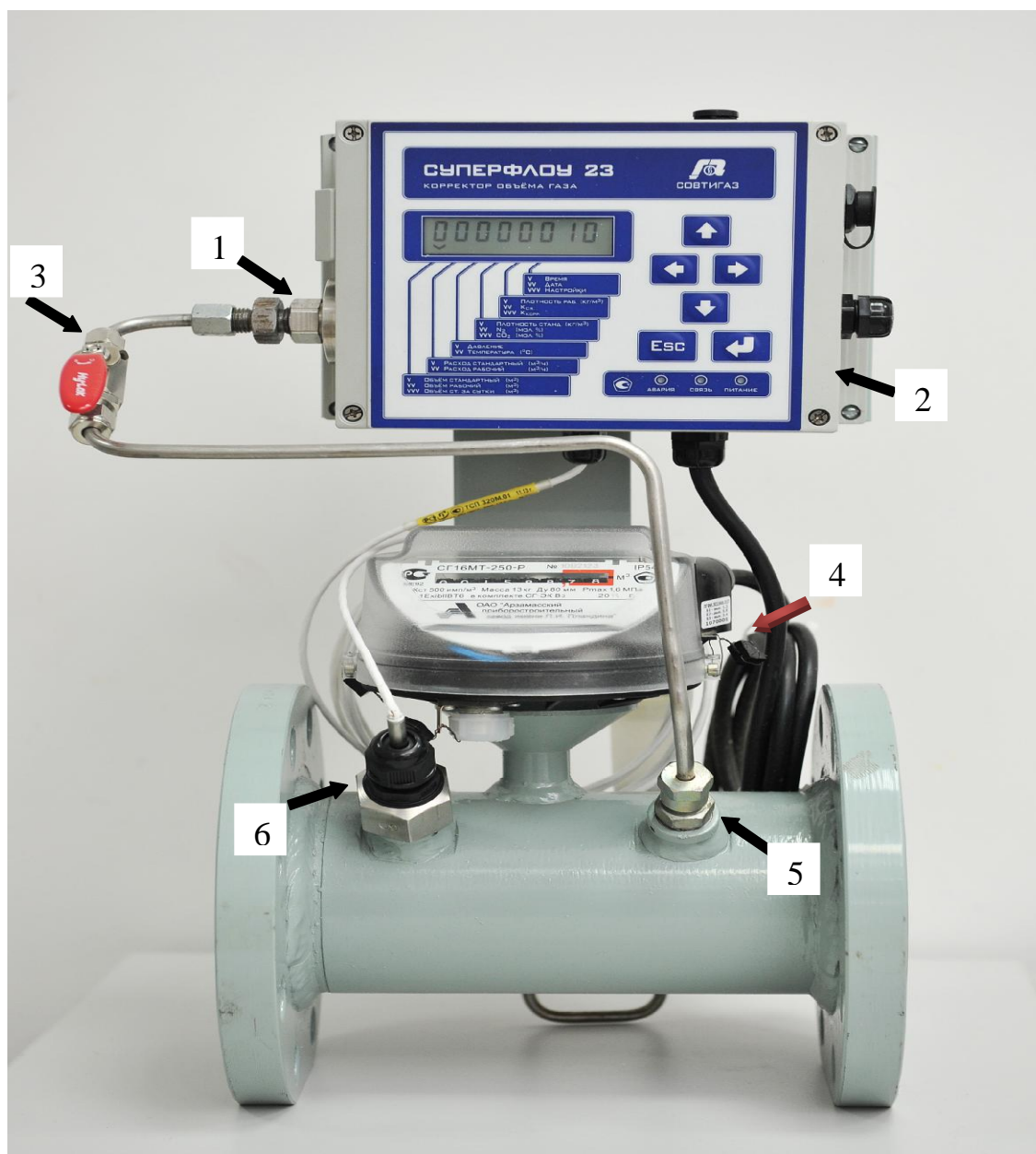
Рисунок 1 - Общий вид и схема пломбирования комплексов измерительных "СГ-Суперфлоу"
