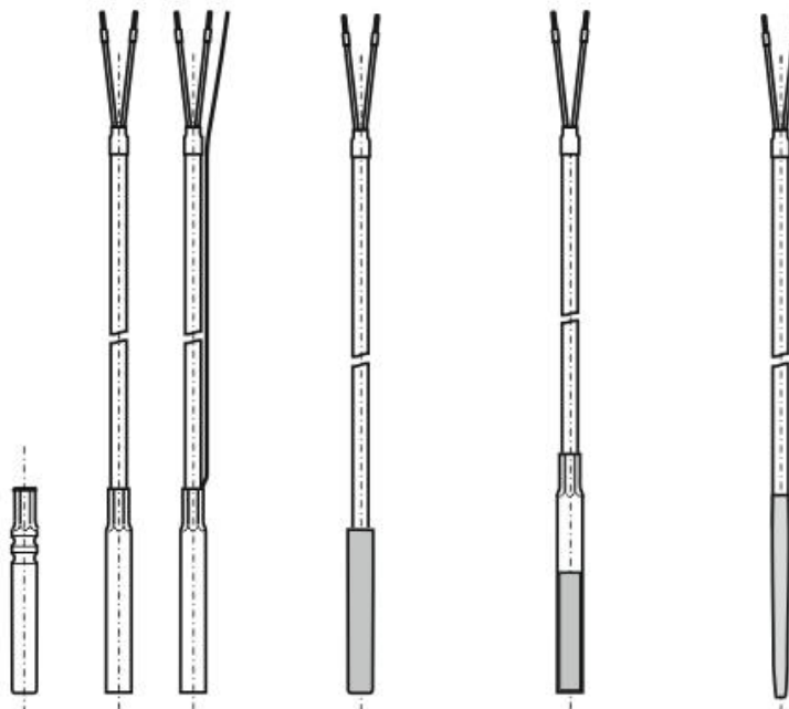
Рисунок 10 - Термопреобразователи модификаций Ruster KF-EXV21A, Ruster KF-EXV21B, Ruster KF-EXV21C, Ruster KF-EXV21FEP, Ruster KEXV21Af, Ruster KEXV21Bf, Ruster KEXV21Cf, Ruster KEXV21FEPf
