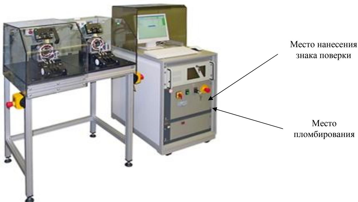
Рисунок 5 - Внешний вид тестеров МТС3-хх с указанием мест пломбирования и нанесения знака поверки
