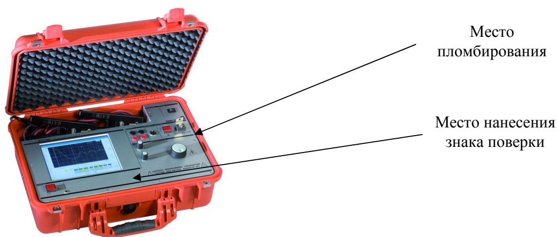
Рисунок 1 - Внешний вид тестеров МТС2-хх компактного исполнения с указанием мест пломбирования и нанесения знака поверки
