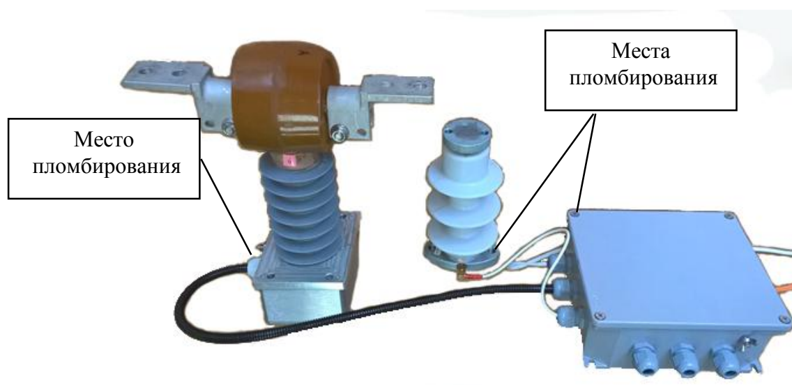
Рисунок 3 - Внешний вид ЦТТН 6(10) -35 кВ опорного исполнения с двумя измерительными узлами для измерения силы тока и напряжения с электронным блоком, выполненным в отдельном корпусе
