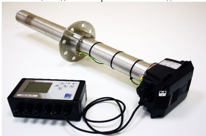
Рисунок 2 - Общий вид анализаторов пыли РСМЕ модели QAL 181
