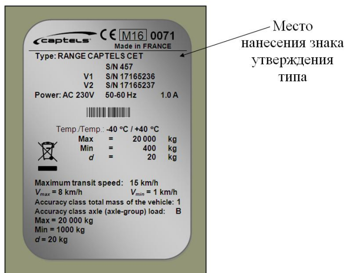
Рисунок 3 - Маркировочная табличка
