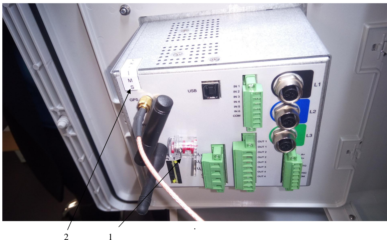
Рисунок 3 - Общий вид счетчика с местами пломбировки изготовителя (1) и поверителя (2)
