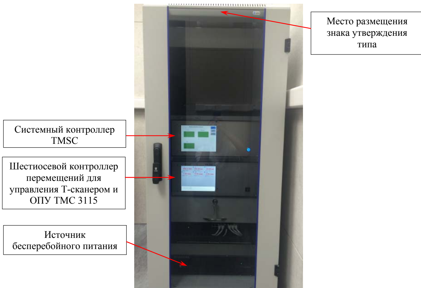
Рисунок 6 - Внешний вид приборной стойки с установленным оборудованием и места размещения знака утверждения типа
