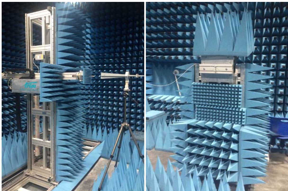
Рисунок 1 - Общий вид конструкции сканера ТМП 04П 5.0 x 2.0 (слева), внешний вид опорно-поворотного устройства ТМП02В 350 (справа)
