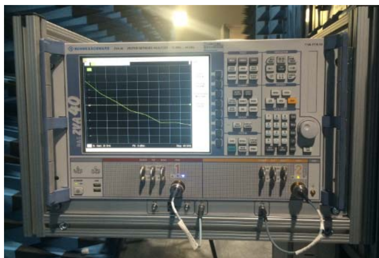
Рисунок 2 - Внешний вид векторного анализатора электрических цепей ZVA 40
