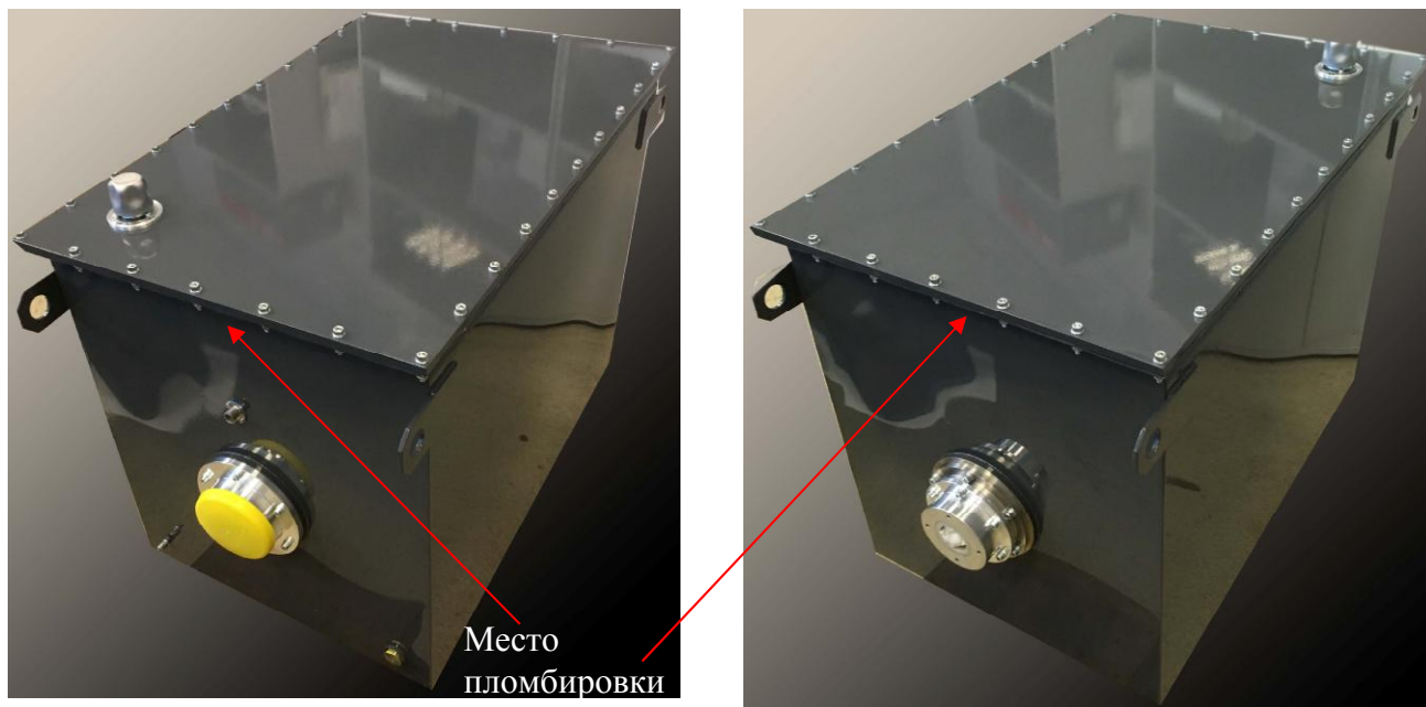
Модификация Экстратестер-250/Э
