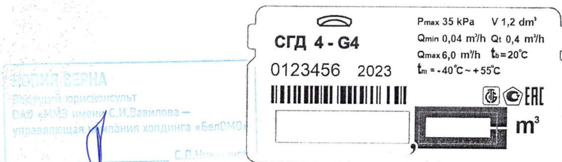
Рисунок 1.2 – Фотография маркировки счетчиков газа диафрагменных СГД 4 (изображение носит иллюстративный характер)
