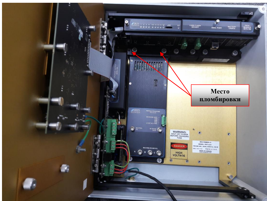
Рисунок 5 - Внутренняя компоновка системы PDTracII
