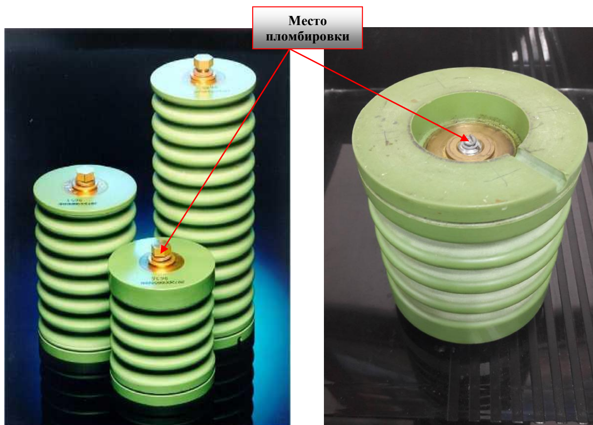
Рисунок 1 - Общий вид датчиков ЧР
