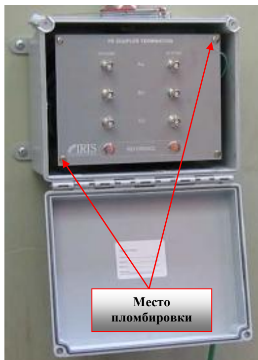
Рисунок 4 – Общий вид соединительной коробки выводов
