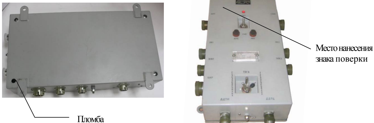
Рисунок 4 - Схема пломбировки от несанкционированного доступа блока БКР-УП
