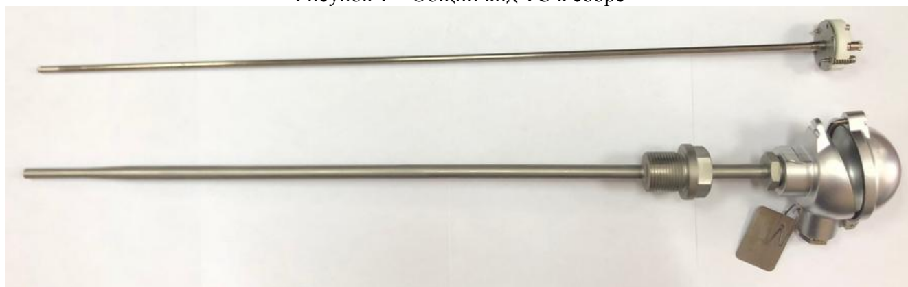
Рисунок 2 – Общий вид ТС в разобранном виде
