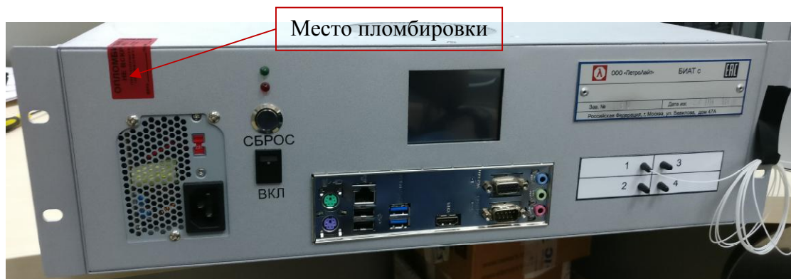
Рисунок 1 – Общий вид блока опроса БИАТ с производства ООО «ПетроЛайт» (лицевая сторона)
