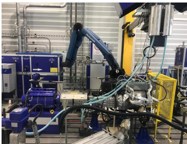
Рисунок 1 – Общий вид стенда
