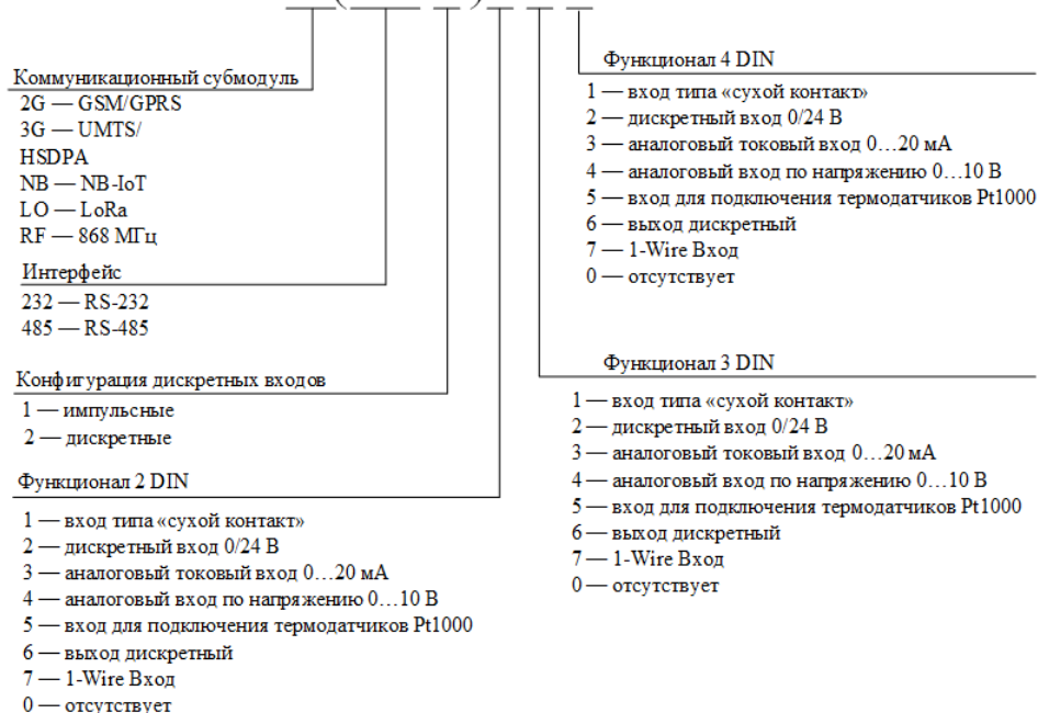
Рисунок 7 – Принцип формирования модификации УСПД M2M Хаб ПЛЮС
