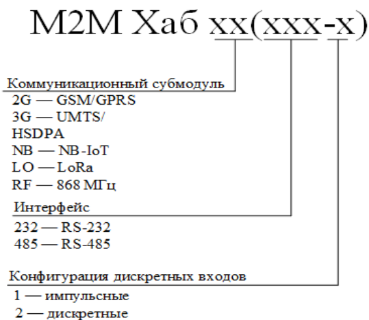
Рисунок 6 – Принцип формирования модификации УСПД M2M Хаб
