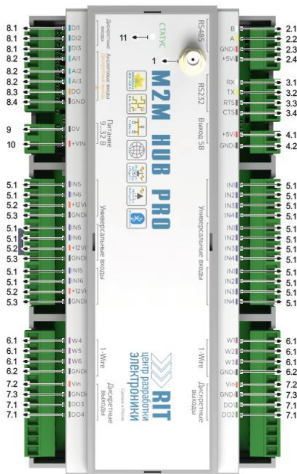
Рисунок 5 – Общий вид M2M Хаб про
