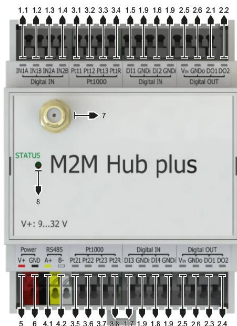
Рисунок 4 – Общий вид M2M Хаб плюс
