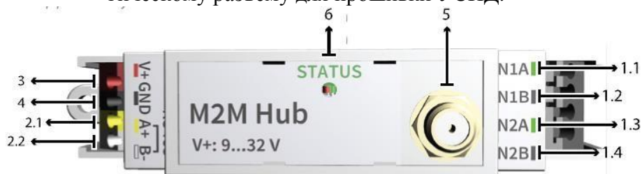
Рисунок 3 – Общий вид M2M Хаб
