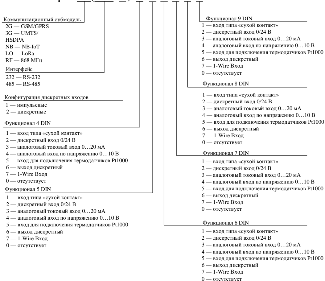
Рисунок 8 – Принцип формирования модификации УСПД M2M Хаб про
