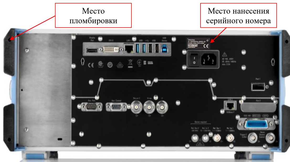
Рис. 2 - Схема пломбировки анализаторов спектра FSV3004, FSVA3004, FSV3007, FSVA3007, FSV3013, FSVA3013, FSV3030, FSVA3030, FSV3044, FSVA3044 от несанкционированного доступа и нанесения серийного номера, идентифицирующего каждый экземпляр СИ
