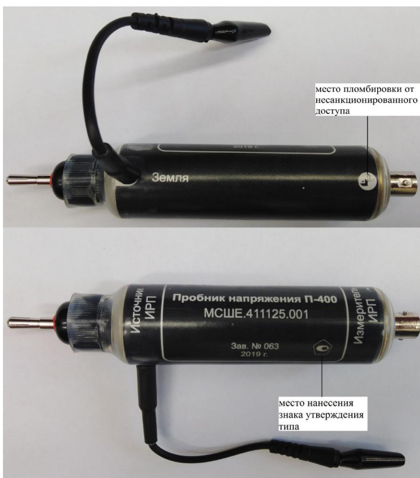
Рисунок 1 – Общий вид пробников П-400
