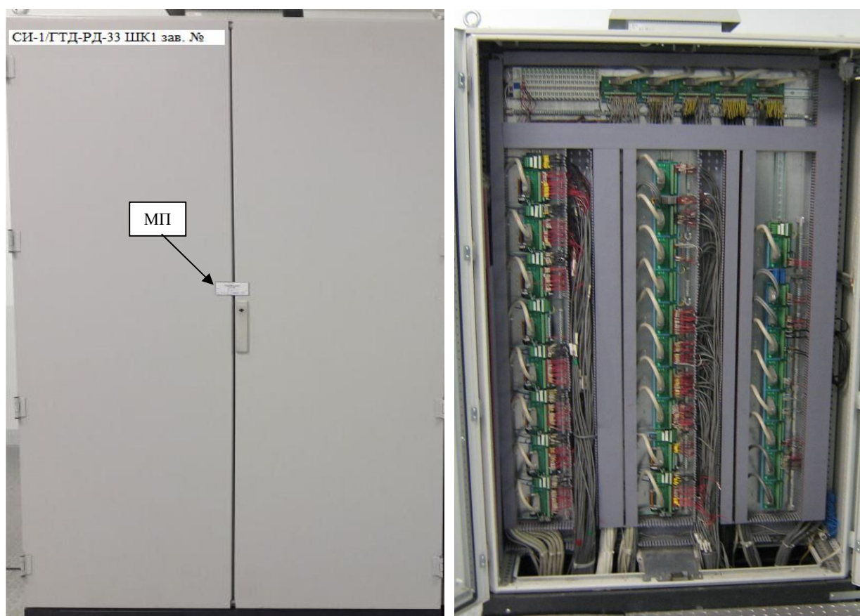
а) – Общий вид вид б) – внутреннее устройство Рисунок 5 – Шкаф ШК1
