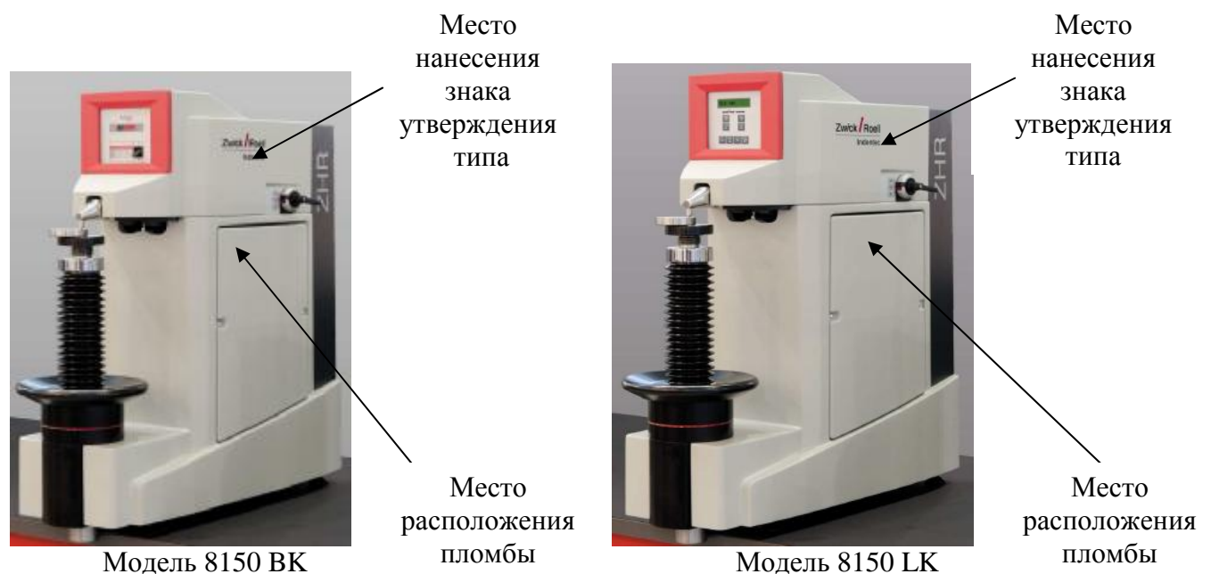
Рисунок 1 – Общий вид твердомеров
