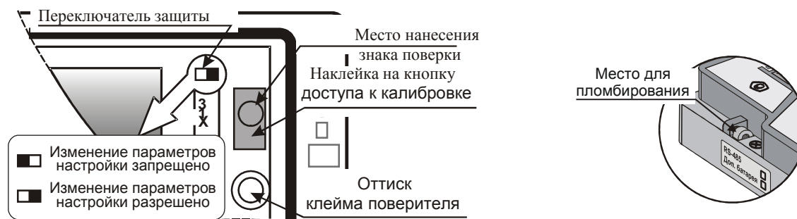
Рисунок 2 – Места пломбирования вычислителя и нанесения знака поверки
