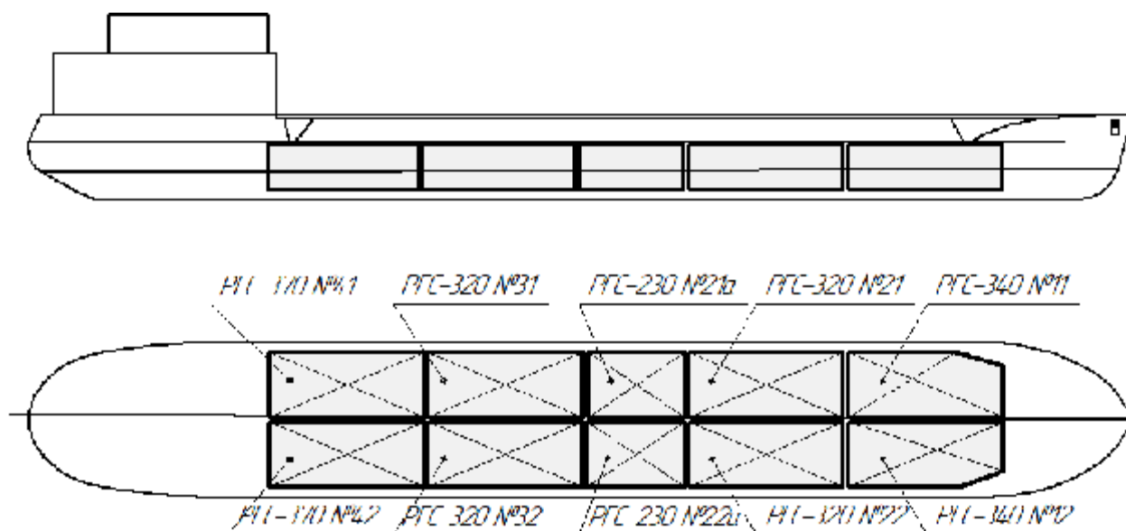
Рисунок 1 – Эскиз общего вида, заводские номера и расположение резервуаров РГС-230, РГС-320, РГС-340, РГС-370
