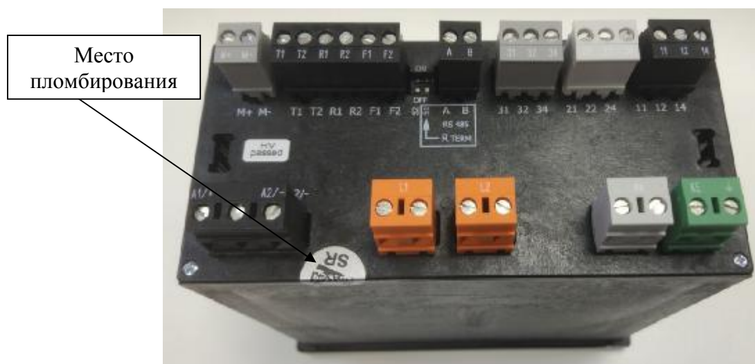
Рисунок 2 - Общий вид сзади устройства контроля сопротивления изоляции ISOMETER IRDH375-435RU (вид сзади) с указанием места пломбирования от несанкционированного доступа с помощью голографической наклейки
