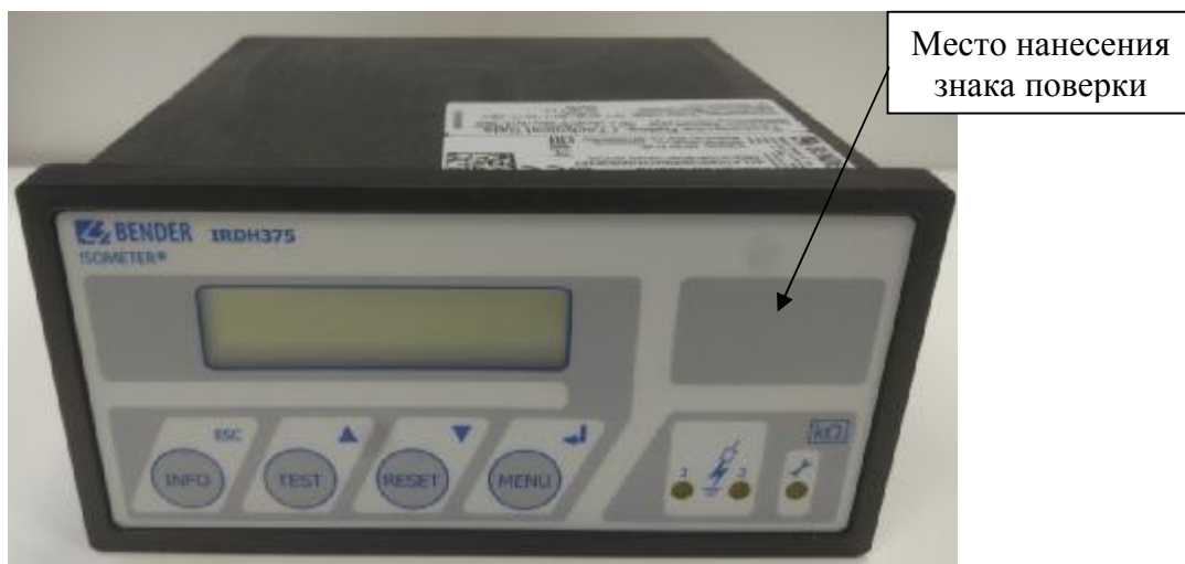
Рисунок 1 - Общий вид спереди устройства контроля сопротивления изоляции ISOMETER IRDH375-435RU с указанием места нанесения знака поверки
