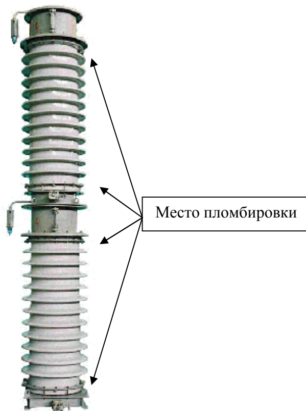
Рисунок 1 – Общий вид средства измерений и схема пломбировки от несанкционированного доступа
