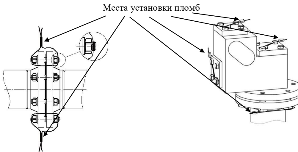
а) фланец калиброванного участка
