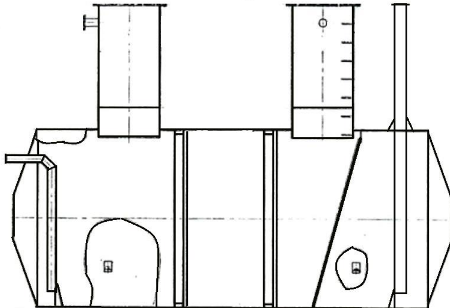
Рисунок 1 – Общий эскиз резервуара
