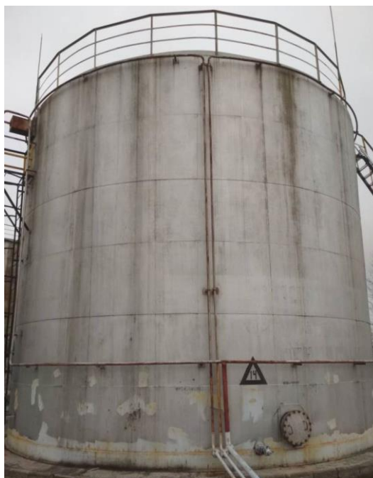
Рисунок 1 – Общий вид резервуара РВСП-700
