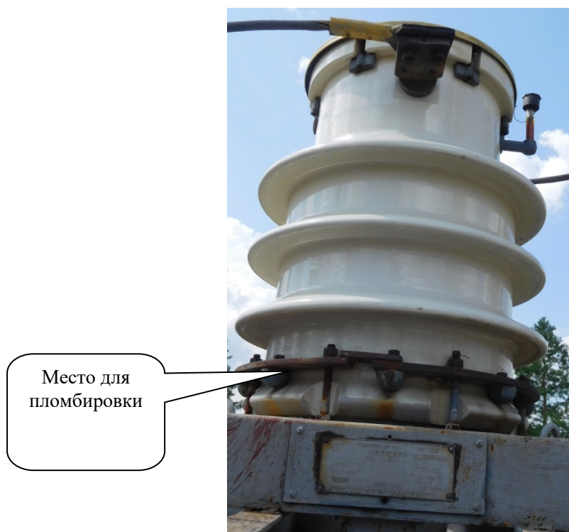
Рисунок 1 – Общий вид трансформатора тока и схема пломбировки ТФ3М 35А-У1
