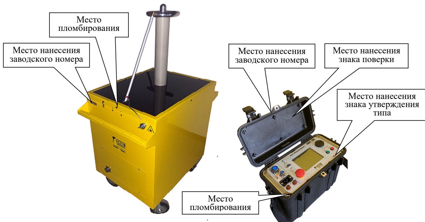
Рисунок 5 – Общий вид аппаратов СКАТ-100Ц, СКАТ-100ЦА с указанием мест пломбовки от несанкционированного доступа, мест нанесения заводского номера, знака поверки и знака утверждения типа
