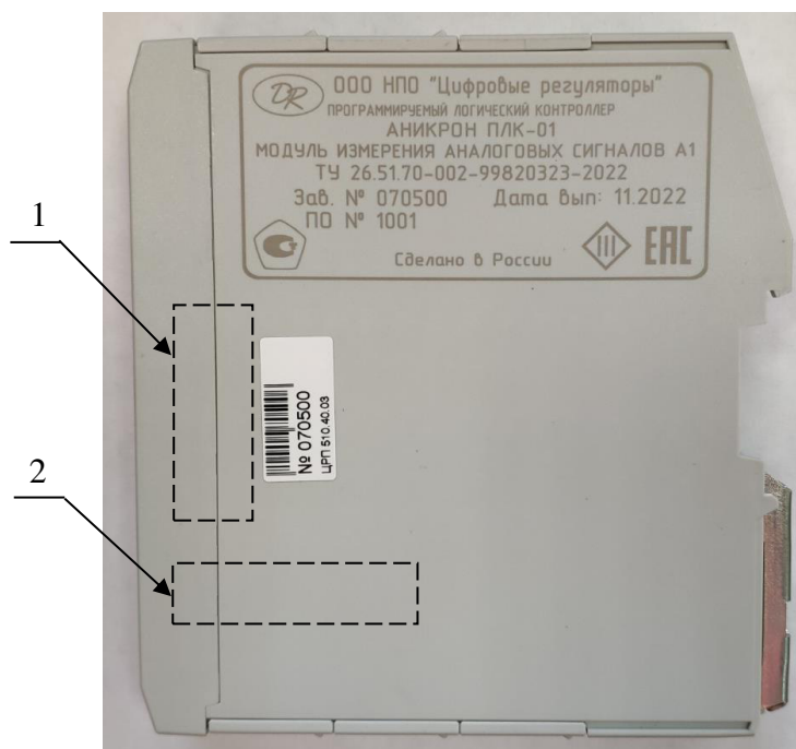
Рисунок 2 – Схема пломбировки Модуля А1 от несанкционированного доступа: 1 – место пломбировки завода-изготовителя; 2 – место нанесения знака поверки.
