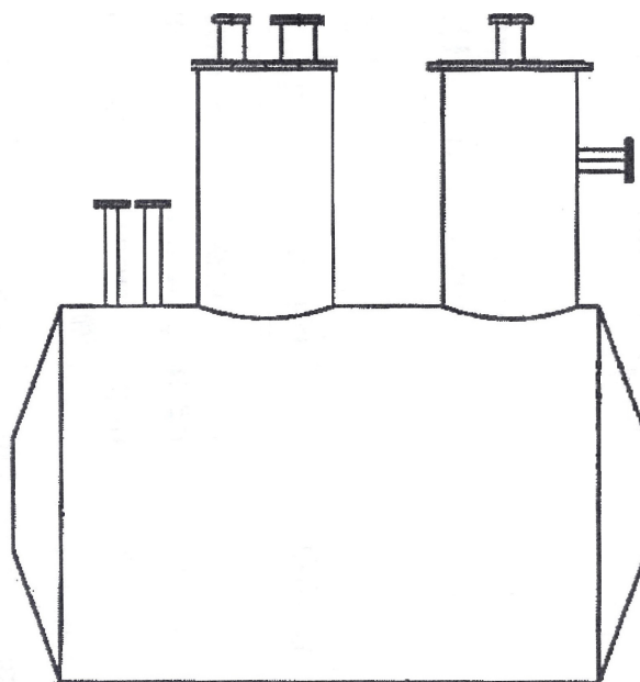
Рисунок 1 – Эскиз резервуара
