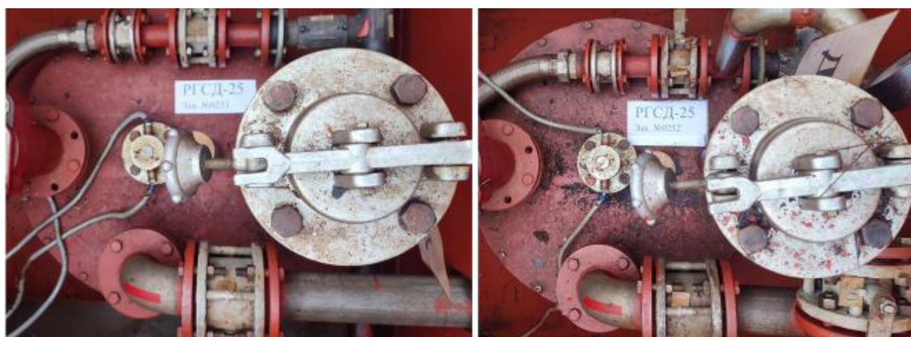
Рисунок 3 – Горловины и измерительные люки резервуаров РГСД-25 зав.№№ 0251, 0252
