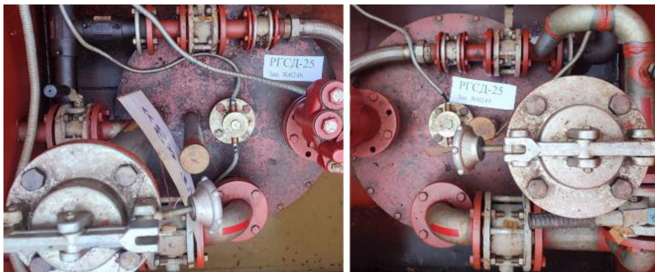
Рисунок 2 – Горловины и измерительные люки резервуаров РГСД-25 зав.№№ 0248, 0249
