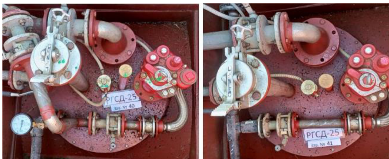
Рисунок 3 – Горловины и измерительные люки резервуаров РГСД-25 зав.№№ 40, 41
