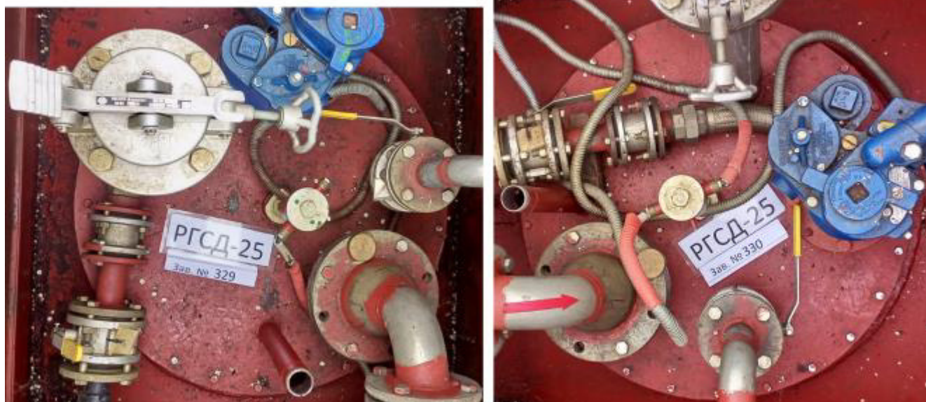
Рисунок 4 – Горловины и измерительные люки резервуаров РГСД-25 зав.№№ 329, 330
